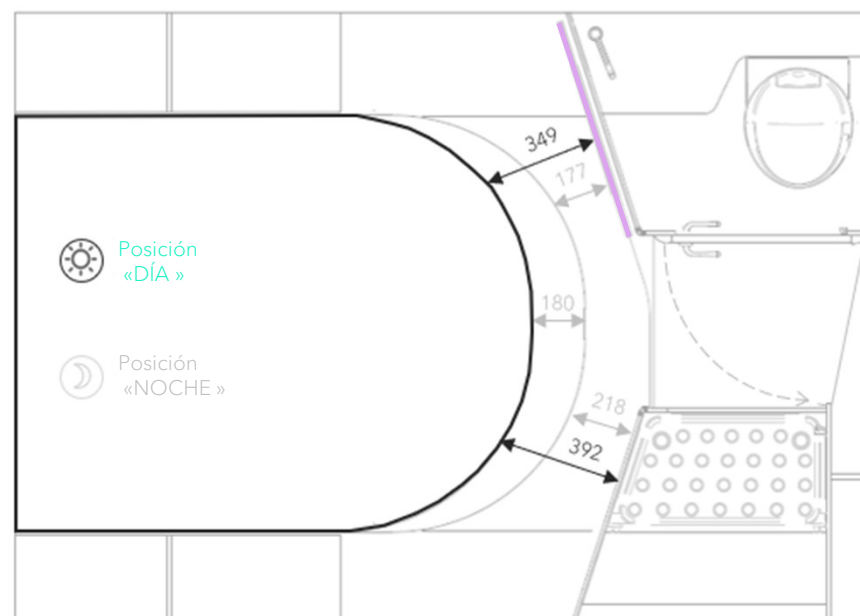
DISTRIBUCIÓN TRADICIONAL CON PUERTA CORREDERA EN LA ZONA DE DESCANSO
